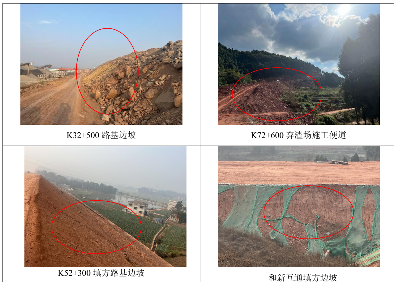
图 5-6 部分边坡无防护区域
